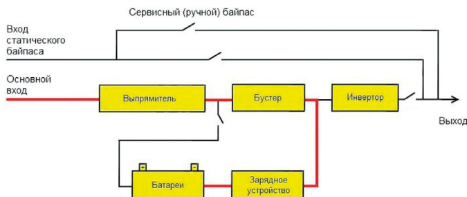
Схема работы в режиме ожидания
