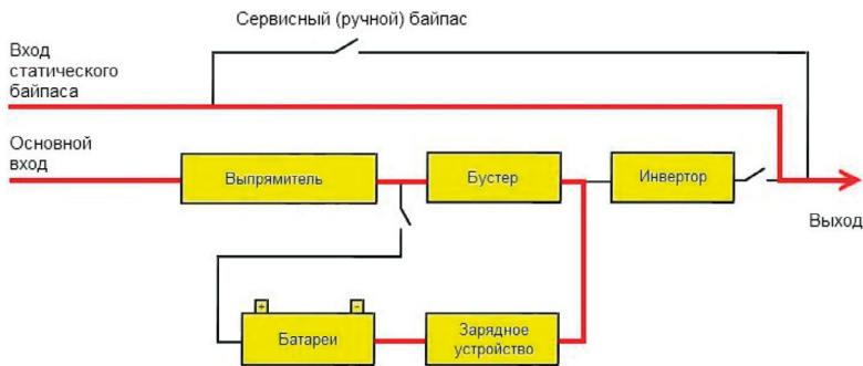
Схема работы в ЭКО режиме
