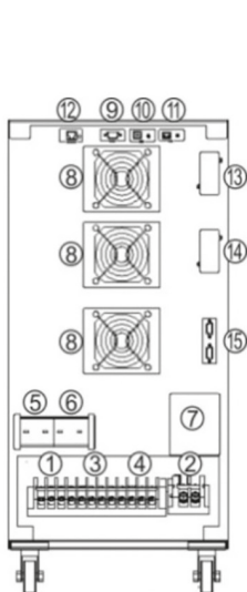
ИБП SW900Pro-T (10 кВА)
