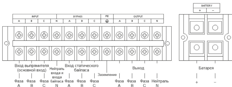
Расположение контактных выводов для ИБП 10кВА
