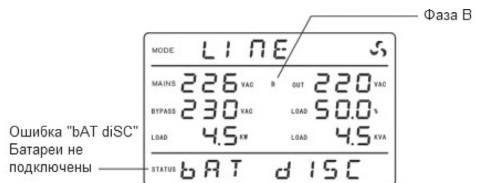
Пример отображения информации по фазе B.
