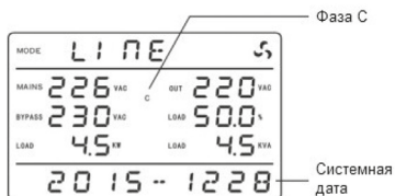
Пример отображения информации по фазе C.
