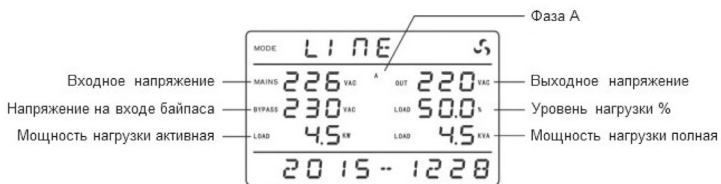
Пример отображения информации по фазе A.
