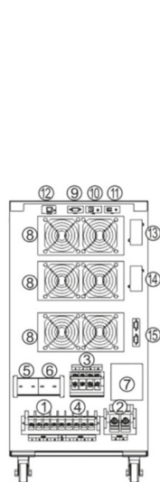
ИБП SW900Pro-T (15/20/30 кВА)
