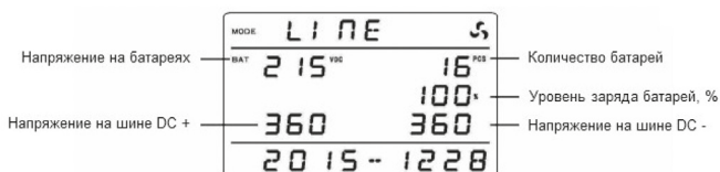
Пример отображения информации по параметрам цепи батарей.
