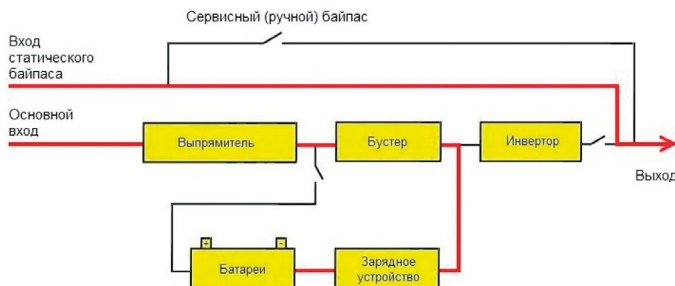
Схема работы в режиме статического байпаса
