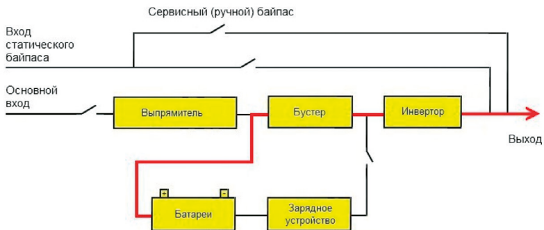
Схема работы в режиме от батарей
