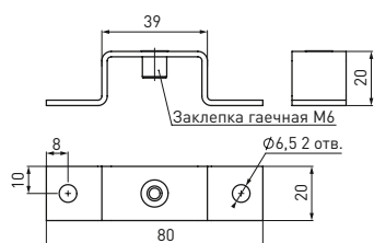
Кронштейн 20 мм
