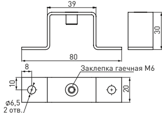
Кронштейн 30 мм
