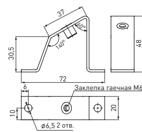
Кронштейн под углом
