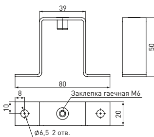
Кронштейн 50 мм
