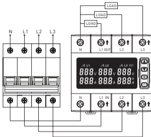
Рисунок 5. Схема подключения реле
