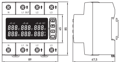
Рисунок 4. Габаритные и установочные размеры изделия
