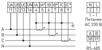
Рисунок 5 – Схема подключения приборов SM-B-96, SM-B-72
