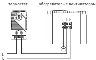
Рис. 2 Подключение обогревателя
