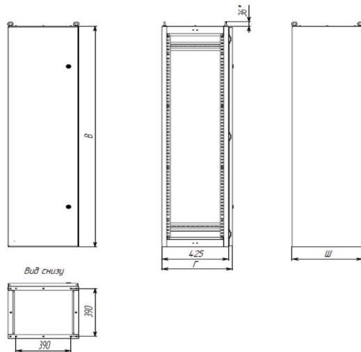
Рис.1 - Общий вид шкафов ВРУ-1 Unit R
